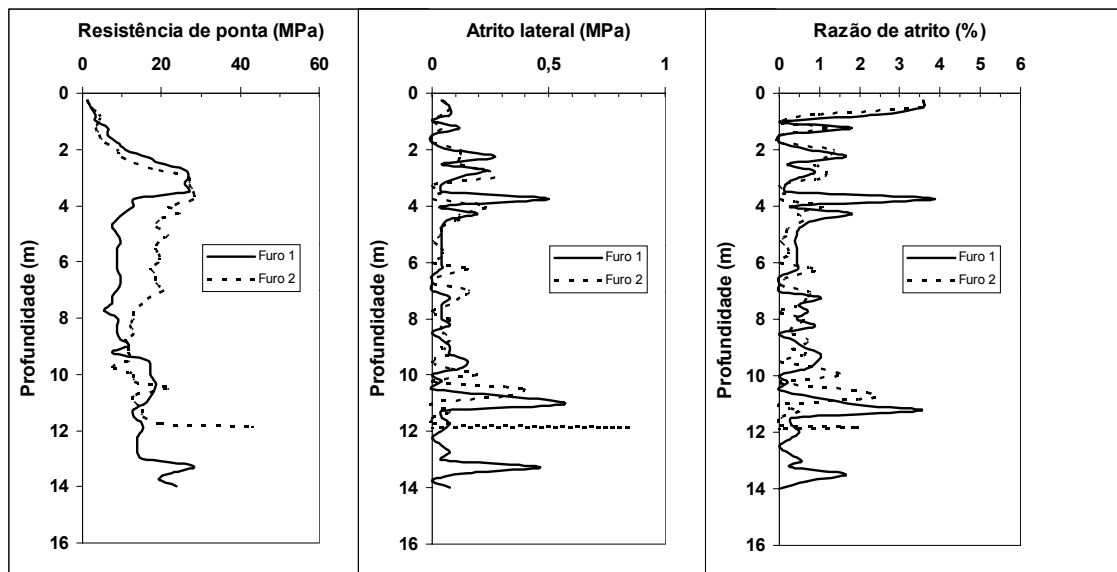
Figura 2 – Resultados de ensaios de cone mecânico - CPT
