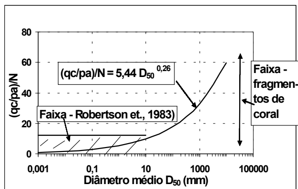
Figura 5 – Variação de qc/N com o diâmetro da partícula (modificado de Robertson et al., 1983)
