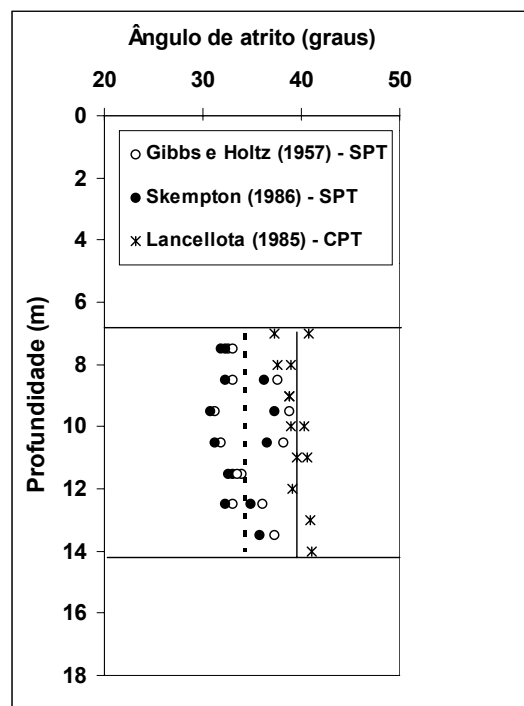
Figura 4 – Variação do ângulo de atrito com a profundidade – Correlação de Meyerhof (1956) em função da densidade relativa
