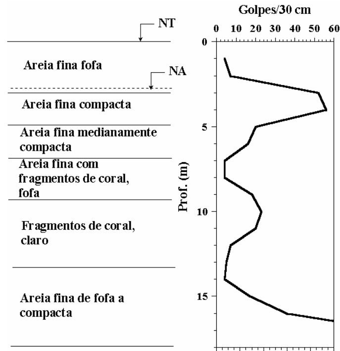
Figura 1 - Perfil geotécnico do subsolo – Sondagem SPT
