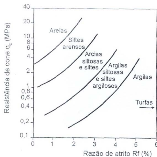
Figura 3 – Ábaco para classificação do tipo de solo sedimentar (Robertson e Campanella, 1983, citado por Schnaid, 2000)
